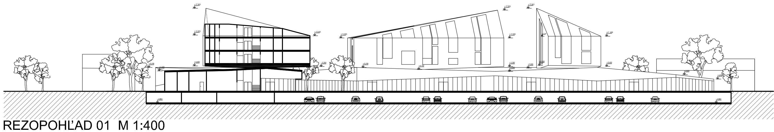
REZOPOHĽAD 01 M 1:400
